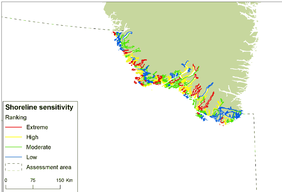
Ilusiliaq 2. Sinerissami killeqarfiup uuliakoornermut malussarissusaa, DMU-ip sinerissami killeqarfimmut nunap assiliaa 2004-imeersoq malillugu. Sinerissami sumiiffiit malussarinnerpaajusut aappaluttumik allassimapput, aammalu malussarinnginnerpaajusut tungujortumik allassimallutik.
