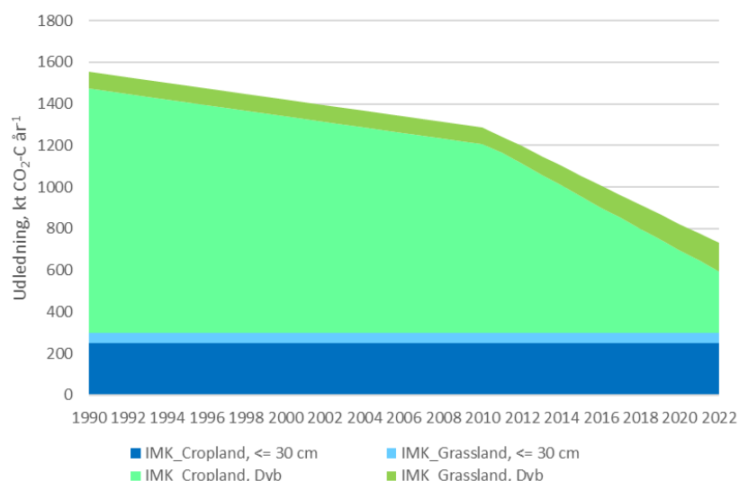
Figur 6 Beregnede CO 2 -udledninger 1990-2022 for de fire forskellige arealklasser opgjort som kt CO 2 -C år -1 .
