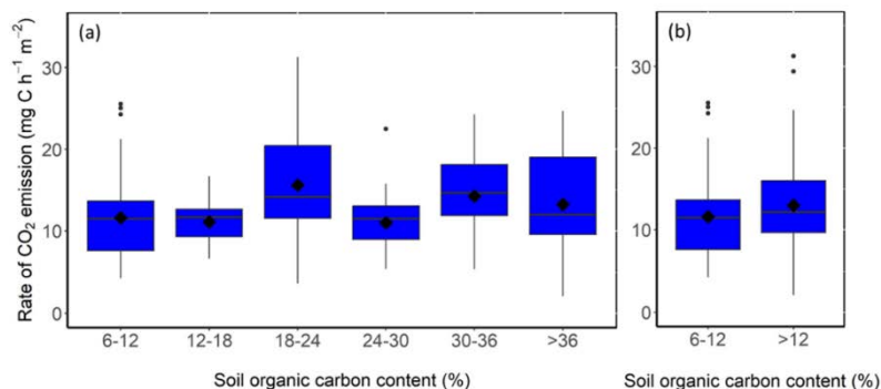
Figur 3 Laboratiormålinger af emissionen af CO 2 -C fra uforstyrrede organiske profiler af topjord (Liang et al., 2024). Data repræsenterer 103 organiske jorder i Danmark, opdelt i klasser med forskelligt organisk kulstof (OC) indhold (a) og samlet for de to klasser med 6-12 % OC og >12 % OC (b).
