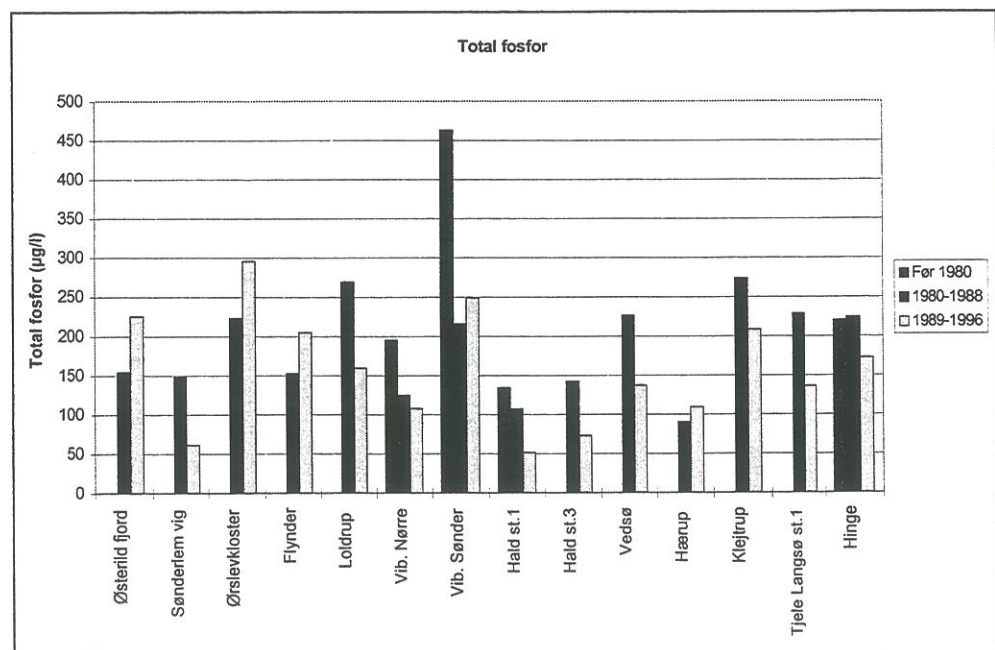
Figur 4.2.1. Udviklingen i sommer gennemsnits koncentrationen af total fosfor i 13 søer i Viborg amt. For søer, hvor der er mere end 1 års målinger indenfor hver tidsperiode er der beregnet en gennemsnitsværdi for perioden.
