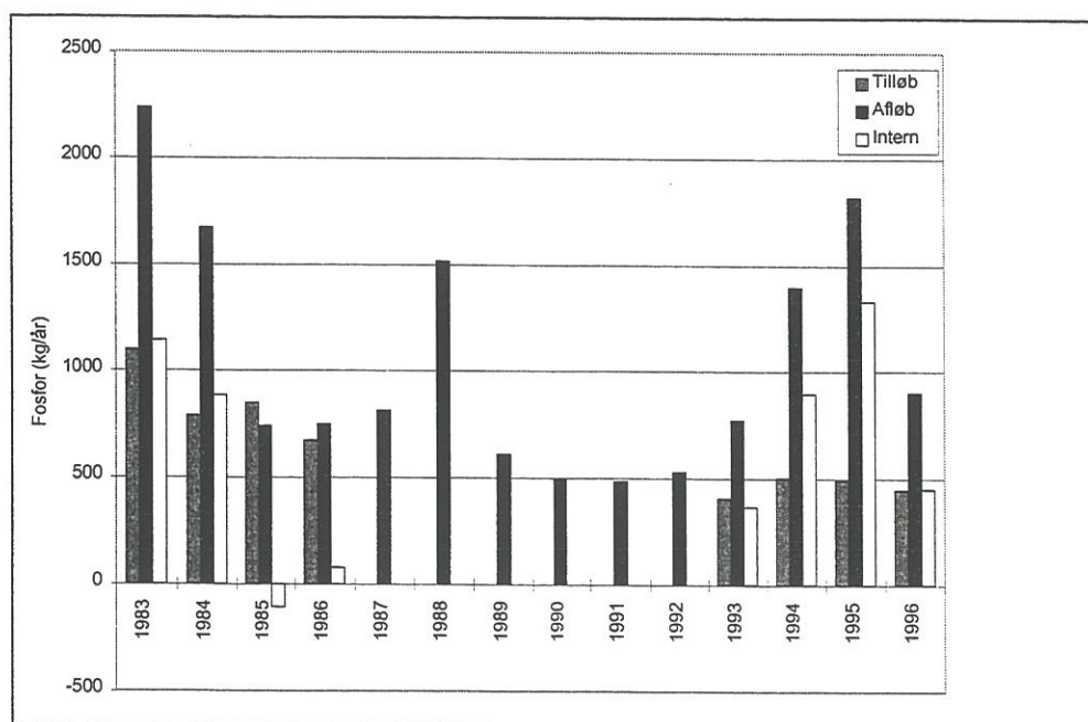
Figur 4.3.6. Massebalance for total fosfor i Klejtrup Sø.
