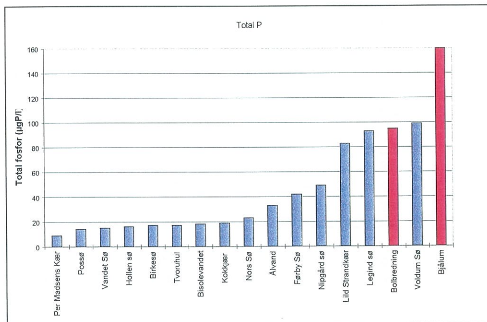
Figur 4.1.1. Vinter koncentration af total fosfor i udvalgte søer i Thy området samt Birke sø, Nipgård sø og Legind sø. Prøverne er udtaget i vinter perioden 1990 - 1996. Målsætningen er ikke opfyldt for Bolbredning og Bjålum.
