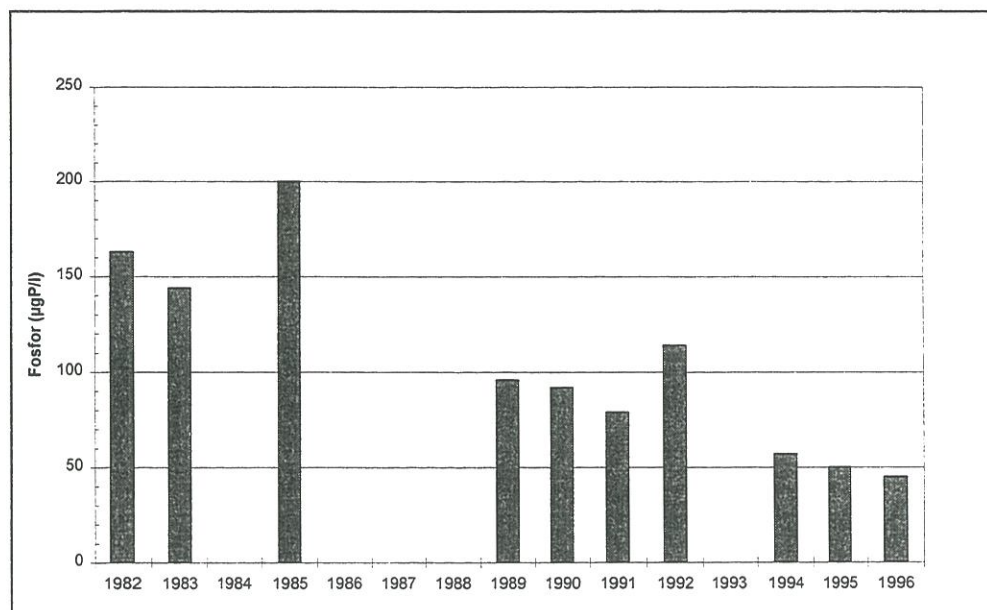
Figur 4.3.3. Udviklingen i tidsvægtet årsmiddelmåling af total-fosfor i epilimnion i Hald Sø.
