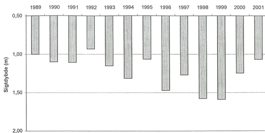
Figur 3.22. Sigtdybden (års gennemsnit) i Kvie Sø 1989-2001.
