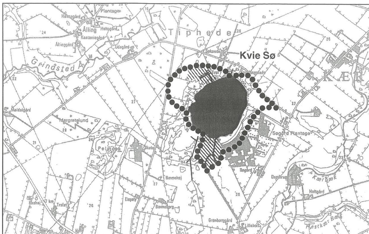
Bilag 2.1. Hydrologiske opland for Kvie Sø. Det skraverede område markerer oplandet for de afskærede dræn.
