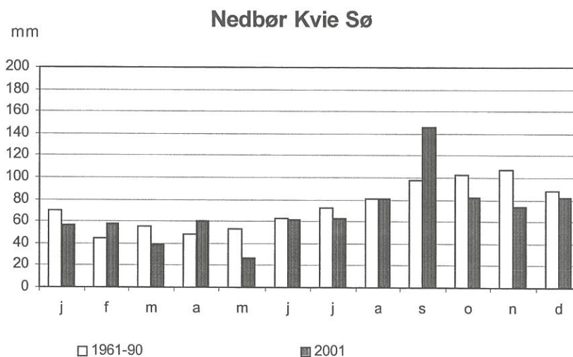
Figur 3.3. Nedbør (mm) ved Kvie Sø i 2001 og som normalværdier for perioden 1961-90. Der er benyttet ukorrigerede griddata for grid 10094.
