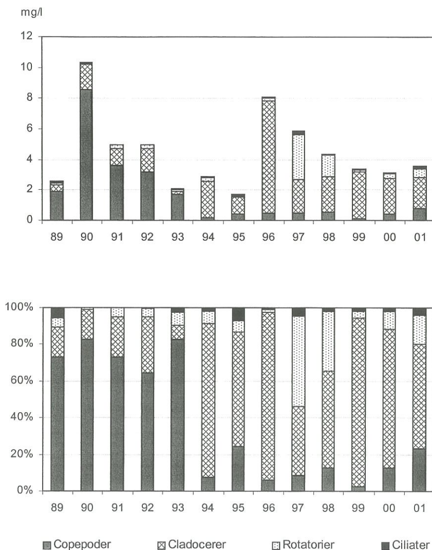
Figur 3.11. Kvie Sø 2001. Dyreplanktonbiomasse og procentvis fordeling på hovedgrupper 1989-2001. Gennemsnit for sommerperioden maj-september.
