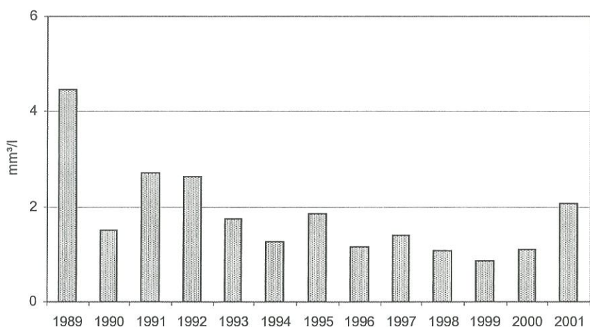
Figur 3.23. Sommergennemsnit (1/5 til 1/10) for biomassen af planteplankton i Kvie Sø, 1989-2001.
