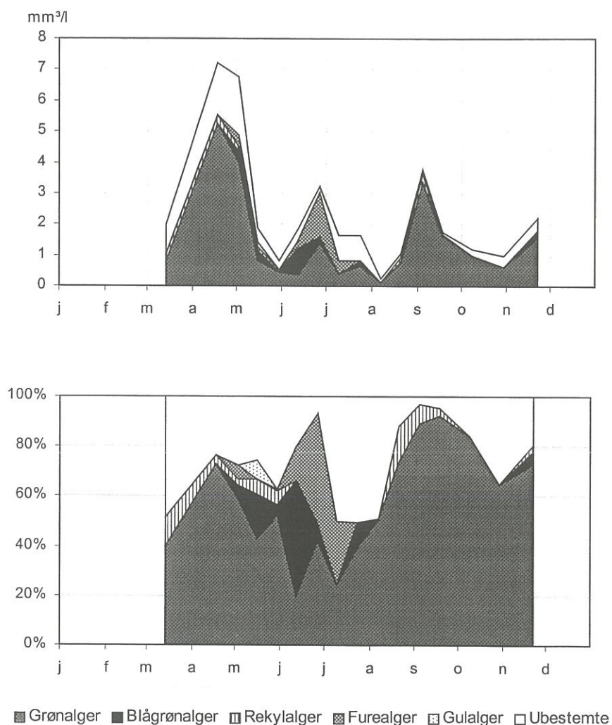
Figur 3.8. Kvie Sø 2001. Planteplankton volumenbiomasse og procentvis fordeling på hovedgrupper.
