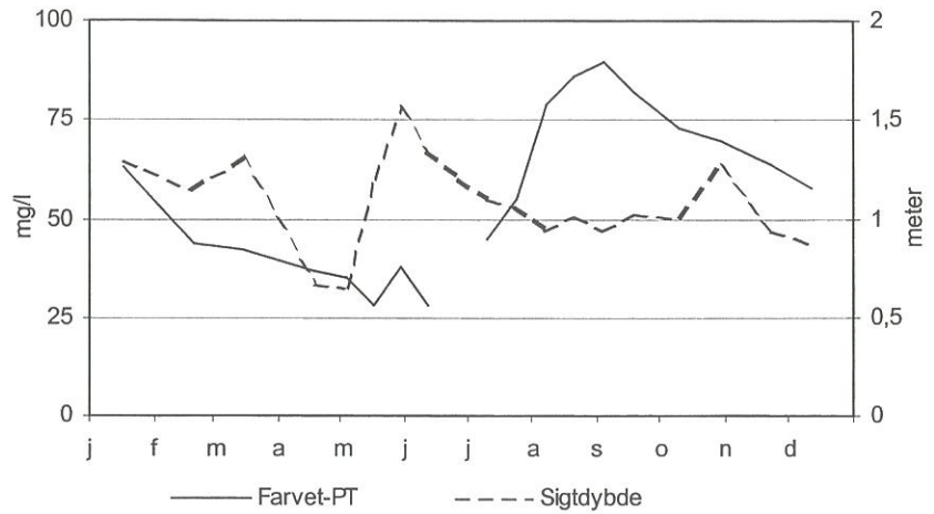
Figur 3.19. Kvie Sø 2001. Forholdet mellem farvetal (mg/l) og sigt dybde (meter).
