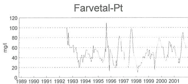
Fig. 3.7. Fysiske og vandkemiske målinger i Kvie Sø 1989 til 2001.
