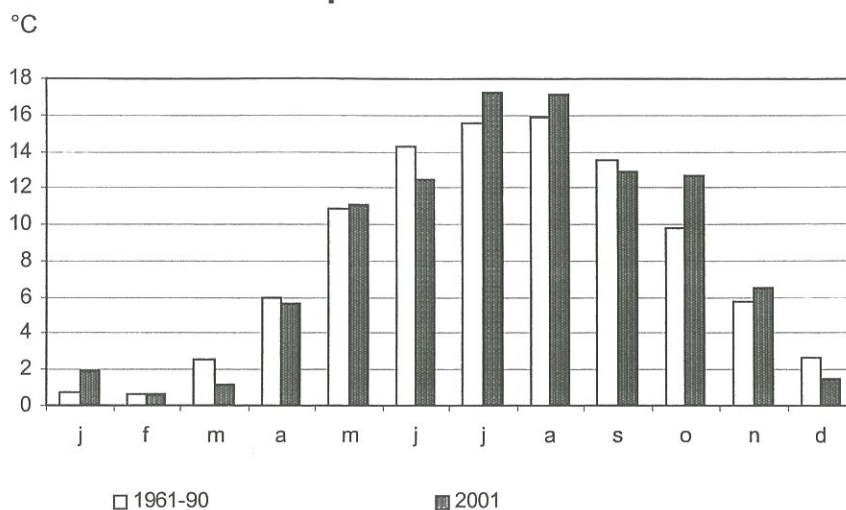
Figur 2.1. Temperatur (°C) ved Holm Sø i 2001 og som normalværdier for perioden 1961-90. Der er benyttet griddata for grid 20008.
