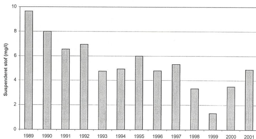
Figur 3.21. Suspenderet stof (årsgennemsnit) i Kvie Sø, 1989-2001.
