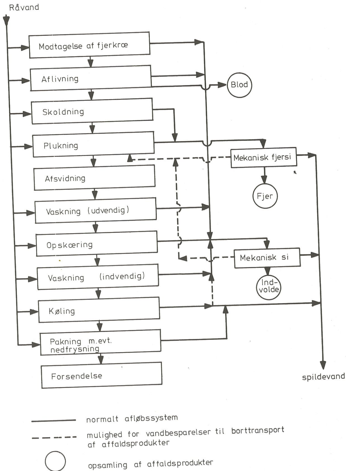
FIG. 1. Enhedsoperationer på fjerkræslagterier.
