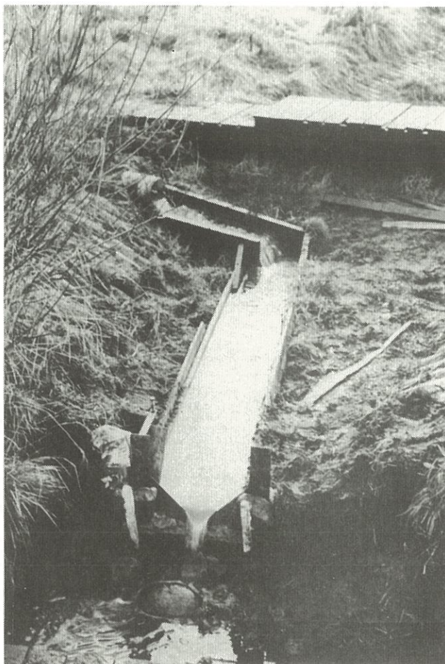
Fig. 5: Opsætning af overfaldsbygværk i afløbsrende.
