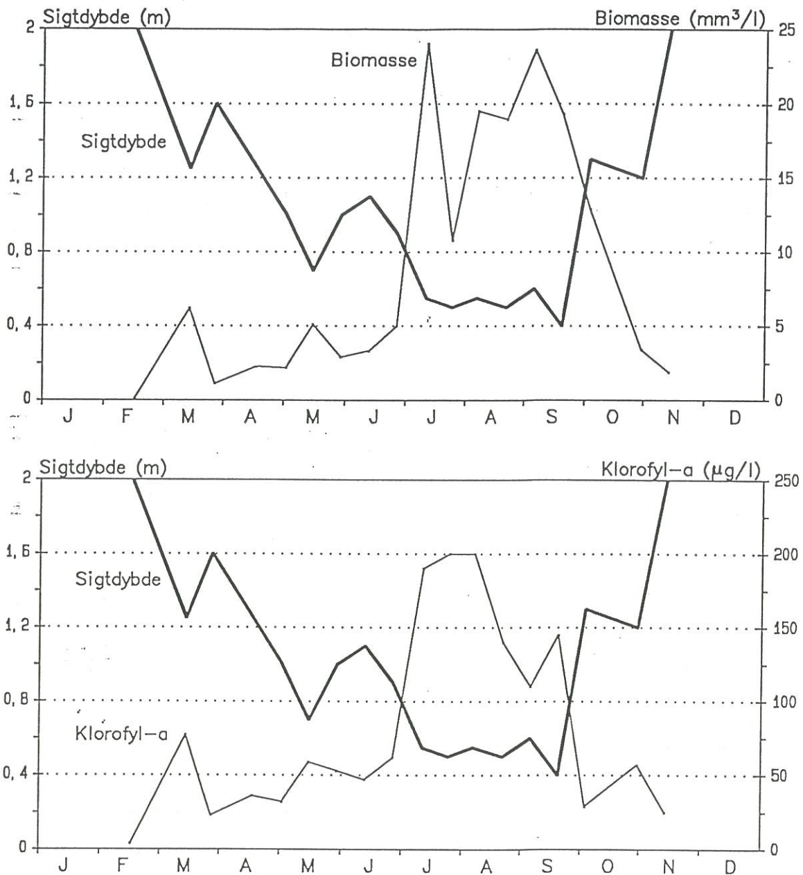
Figur 11. Oversigt over variationen af sigtdybden i Fuglesø 1995. Til sammenligning er vist variationen af planteplanktonbiomassen (øverst) og variationen af klorofyl-a koncentrationen (nederst).
