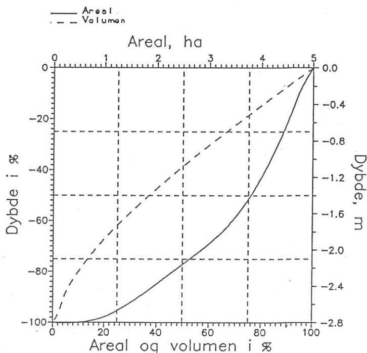
Figur 1. Hypsograf og volumenkurve for Fuglesø, angivet ved vandspejlskote 6,02 m o. DNN. Data efter (Frederiksborg Amt, 1995).
