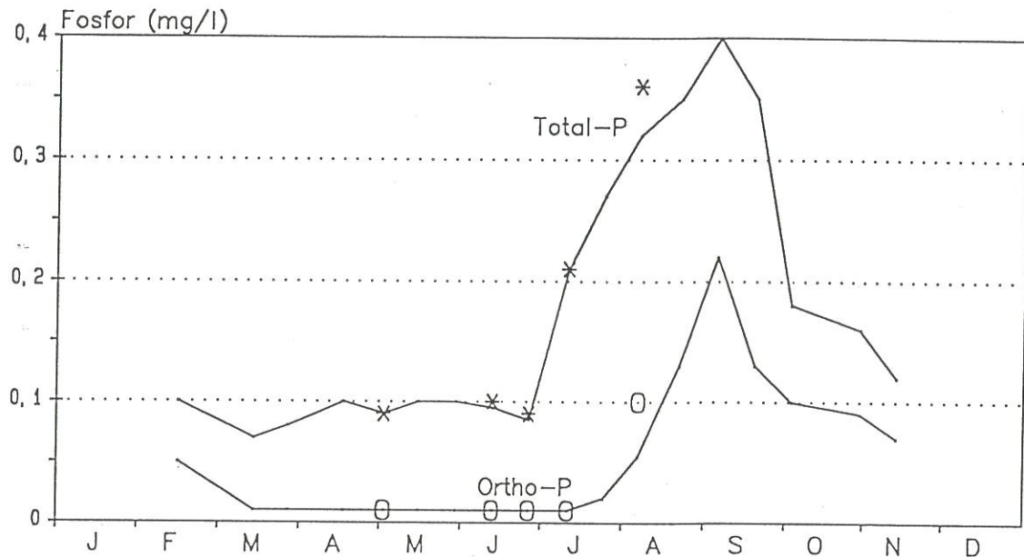
Figur 15. Oversigt over variationen af vandets indhold af fosfor i Fuglesø 1995. Hypolimnion: * = Total-P, o = PO 4 -P.
