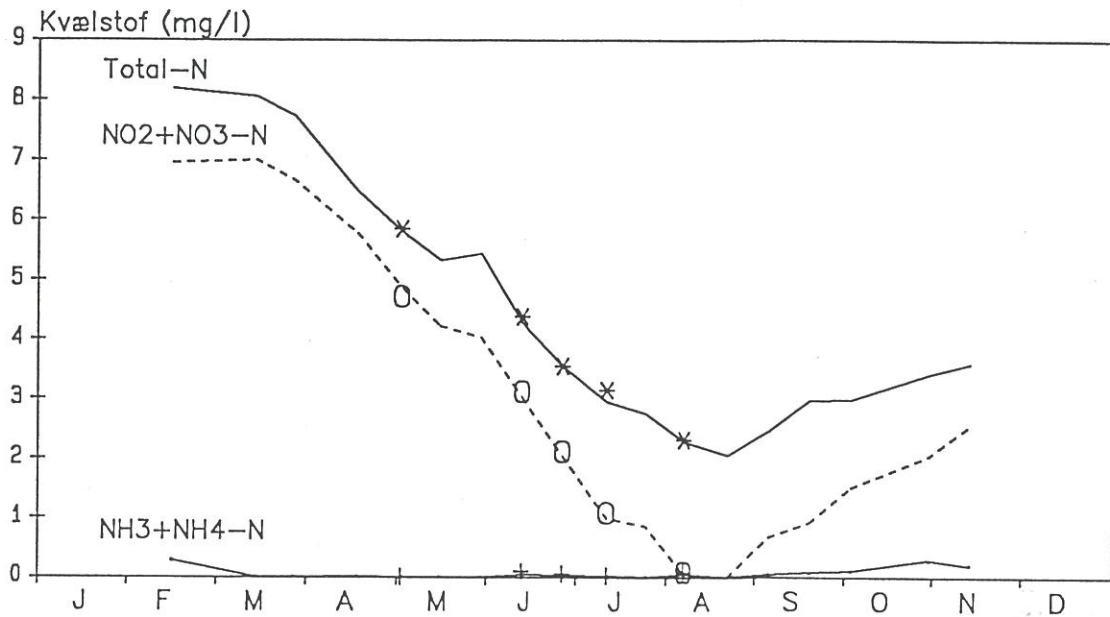
Figur 14. Oversigt over variationen af kvælstof i Fuglesø 1995. Hypolimnion: * = Total-N, o = NO 2 +NO 3 -N, + = NH 3 +NH 4 -N
