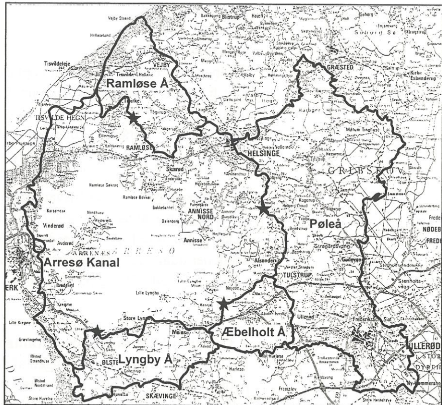
Figur 3.1 Kort over Arresø opland med ★-markering af vandløbsstationer.
