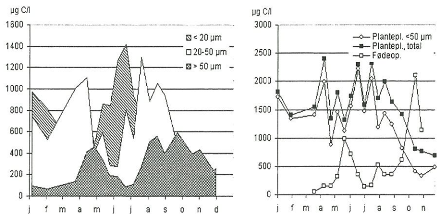
Figur 5.12 Årstidsvariation i planteplanktons størrelsesfordeling (tv) og i dyreplanktonets fødeoptagelse i Arresø 1999 (th).
