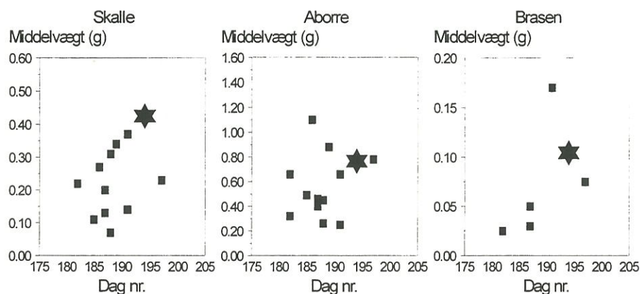
Figur 5.13 Middelvægten af skalle- og aborre- og brasenynglen på undersøgelsestidspunktet i Arresø juli 1999 (stjerne) sammenlignet med årets øvrige undersøgelser (sort markering) og tidligere undersøgte danske søer.
