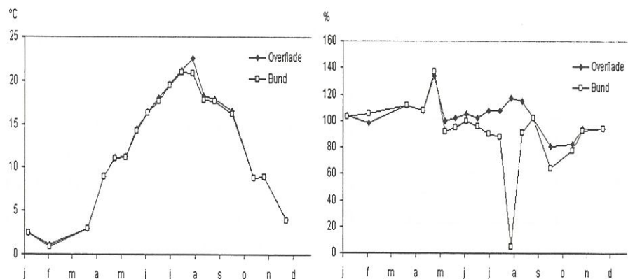
Figur 5.3 Temperatur (tv) og iltprocent (th) i Arresø 1999.
