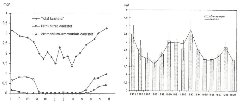
Figur 5.2 Årstidsvariation i kvælstof i Arresø 1999 (tv) og udvikling i sommergennemsnit af total kvælstof 1985-99 (th). Lodrette streger angiver 25 og 75% kvartiler.
