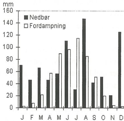
Figur 4.1 Nedbør og fordampning i Arresø 1999
