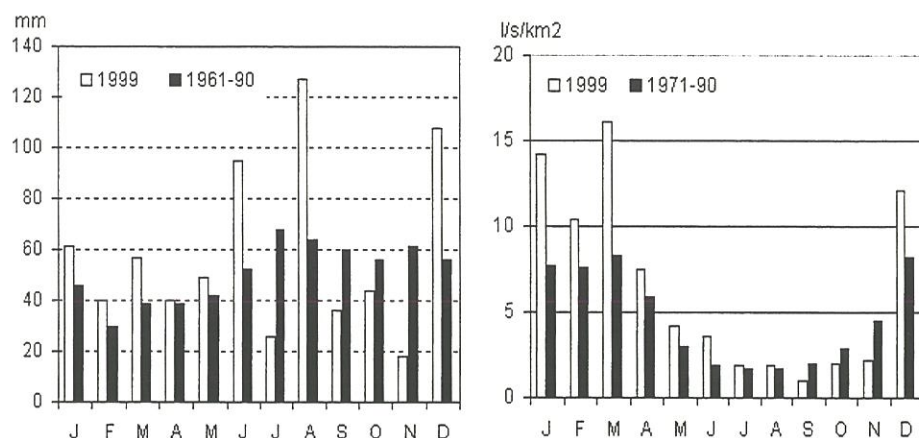
Figur 2.2 Nedbør i det østlige Sjælland. Månedsværdier for 1999 samt normalværdier for perioden 1961-90 (tv). Månedsmiddelfafstrømning i Havelse Å, 1999, samt normalværdier for perioden 1971-90 (th).
