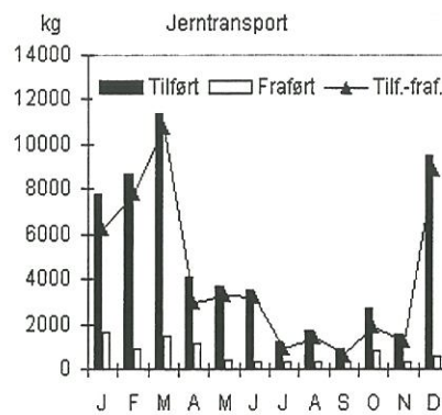
Figur 4.8 Til- og fraførte jernmængder (tv) og jernbalance (th) i Arresø 1999. Alle værdier er i kg.
